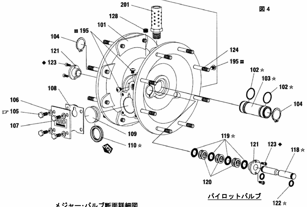
メジャー・バルブ断面詳細図
