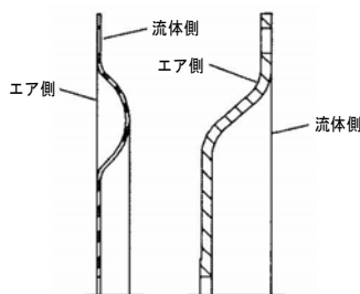
ダイヤフラムの断面図 (頁 5 の図 3 を参照)
