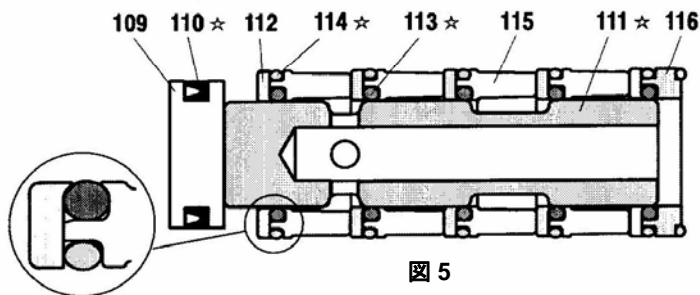
メジャー・バルブ断面詳細図
